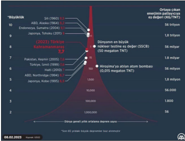
Şekil 1: Son Yüzyılda Dünyada Yaşanan Büyük Depremler
